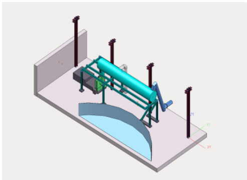
Auf dem CAD importierte Massaufnahme
